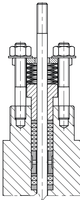
填料函 (石墨) 符合TA-Luft标准
