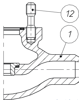
焊接连接阀体 (BW型)
