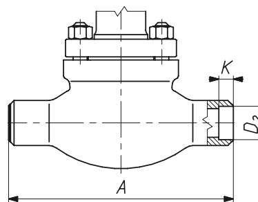
阀体焊接SW型(DN15~50)
