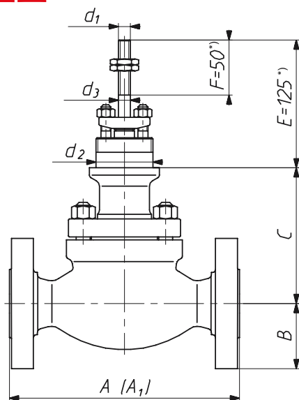
法兰连接控制阀 尺寸E指阀关闭时*E=180mm 执行机构P/R 1000
