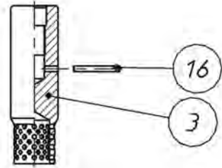
排孔型阀塞
