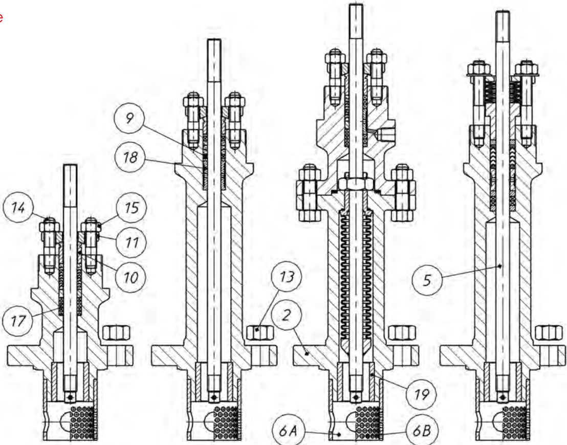
标准型阀盖 PTFE-V形填料
